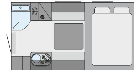
Inneneinrichtung TRAIL/BOX 280
