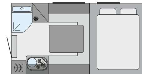
Inneneinrichtung TRAIL/BOX 220
