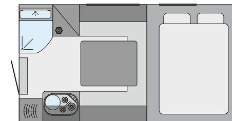
Aménagement intérieur TRAIL/BOX 230
