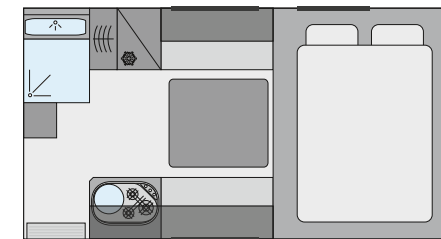
Aménagement intérieur TRAIL/BOX 280S
