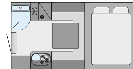
Aménagement intérieur TRAIL/BOX 260
