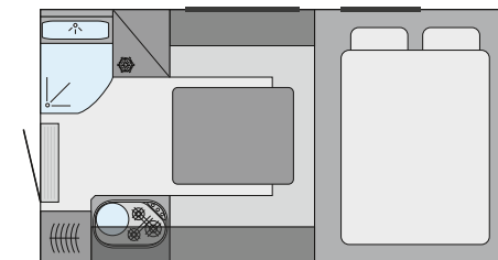
Aménagement intérieur TRAIL/BOX 250
