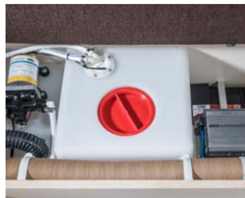
96 Liter-Frischwassertank (außer Trail/Box 200)
